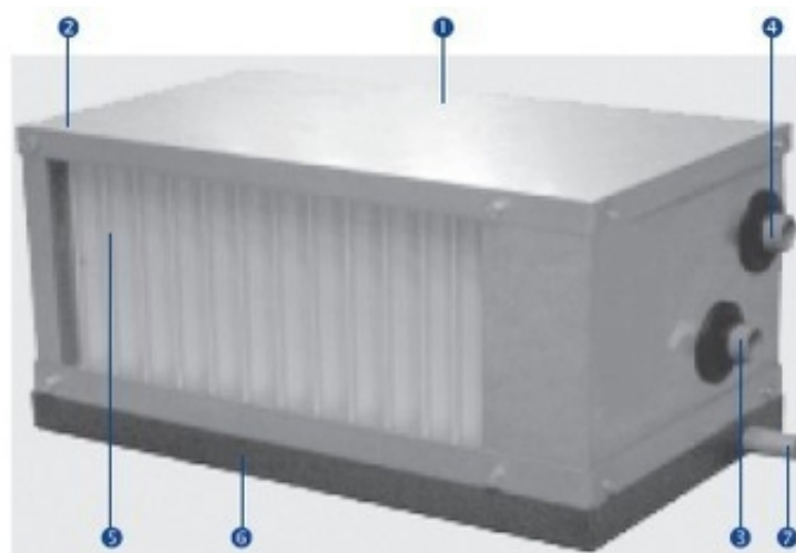
1 корпус, 2 охладитель, 3 подвод хладагента, 4 отвод хладагента, 5 каплеуловитель, 6 ванна для сбора конденсата, 7 отвод конденсата
